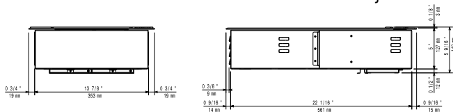
Zij aanzicht
